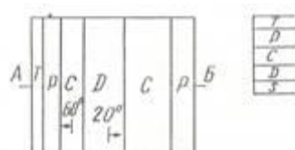
Рис. 9. Геологическая карта и стратиграфическая колонка
