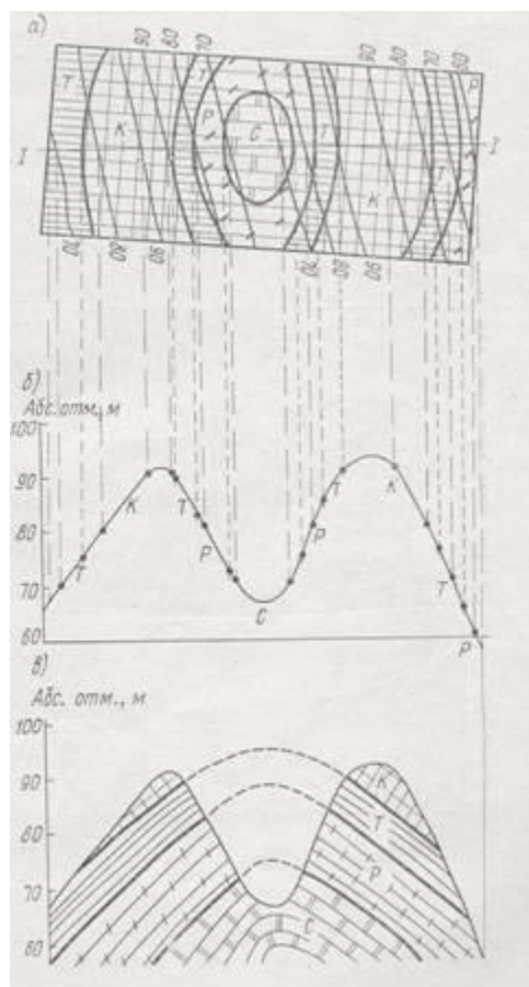
Рис. 8. Пример построения геологического разреза по фрагменту геологической карты 1:1,к с неровной поверхностью рельефа
