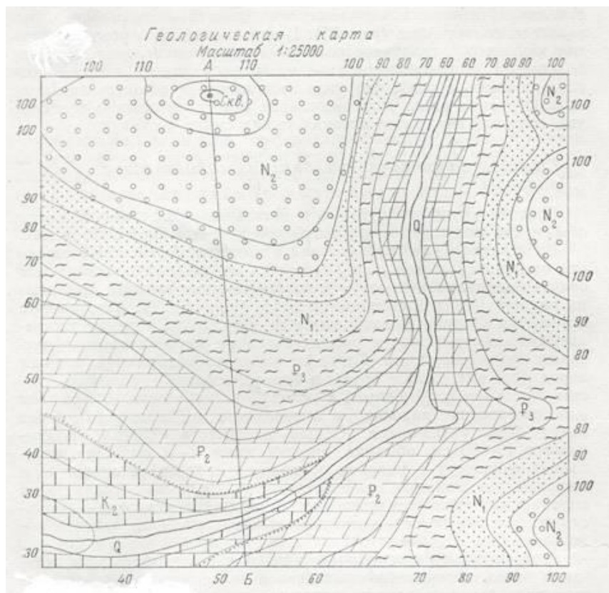
Рис. 1. Геологическая карта участка на топографической основе с горизонтальным залеганием слоев (к зад.2)
