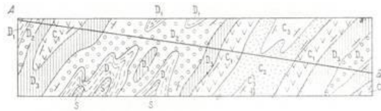
Рис. 11. Фрагмент геологической карты для района со складчатым залеганием горных пород.
