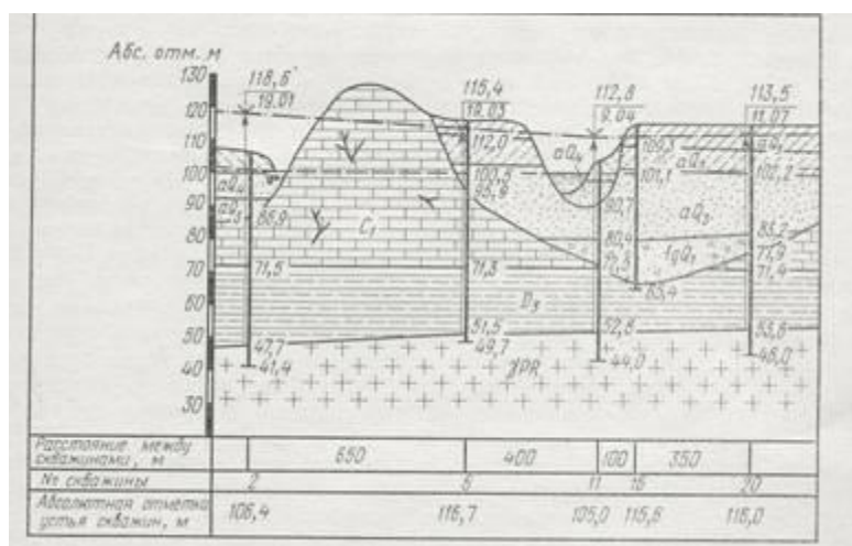
Рис.19. Геологический разрез по линии V-V(на рис. 11)
