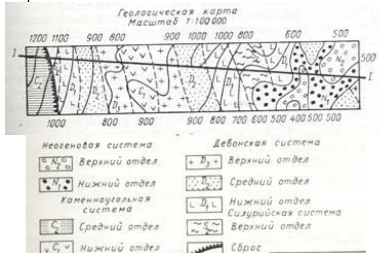
Рис. 14. Геологическая карта
