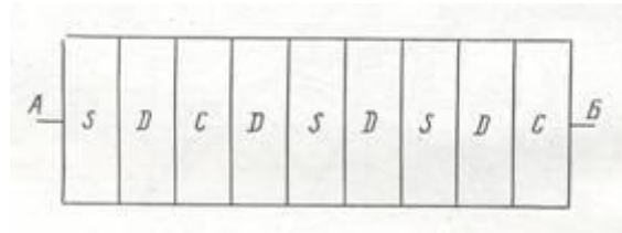
Рис. 9. Геологическая карта участка
