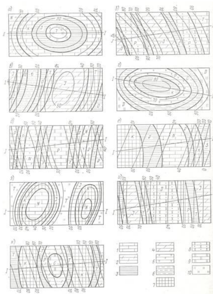
Рис. 7. Фрагменты геологических карт на топографической основе масштаба 1:2000 на участки с неровной поверхностью (к зад.8)
