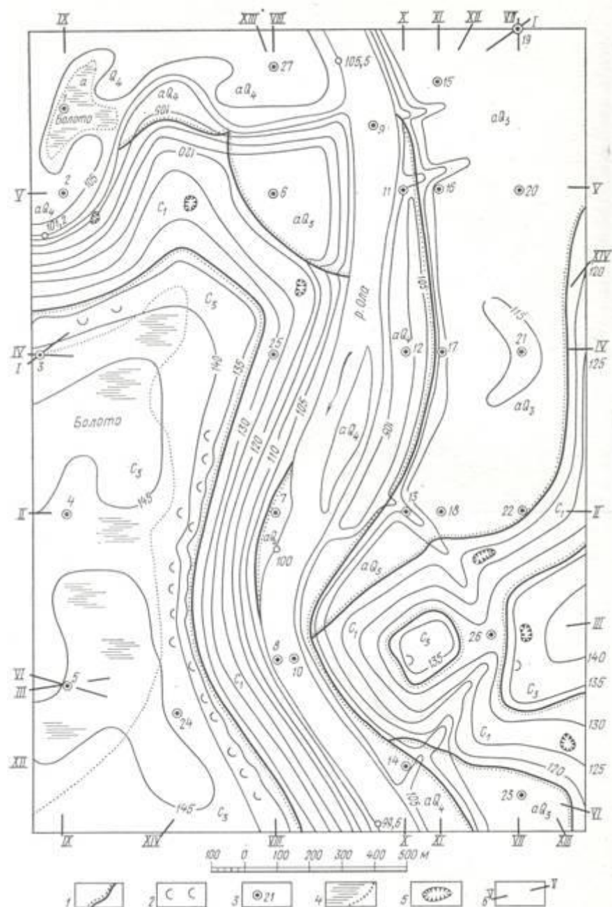
Рис. 16. Геологическая карта:
