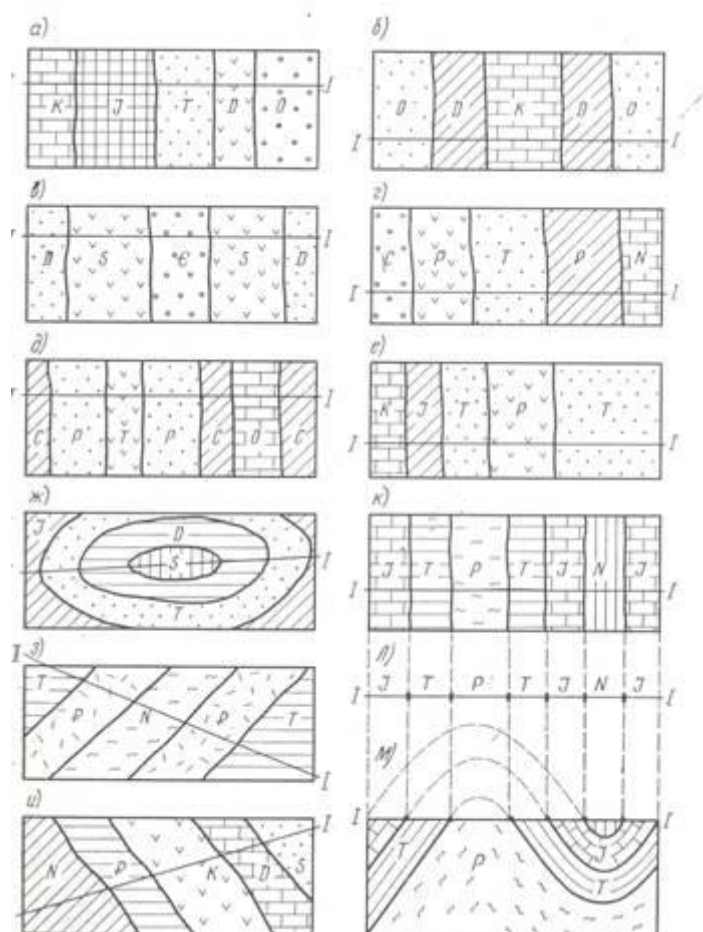
Рис.6. Фрагменты геологических карт на участки с примерно горизонтальной поверхностью рельефа (к зад.7)
