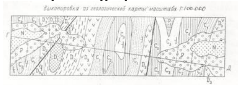
Рис. 13. Фрагмент геологической карты для района со складчатым залеганием горных пород, осложненным сбросами
