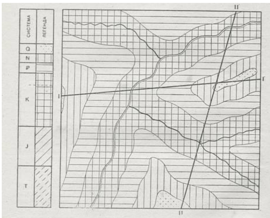
Рис. 2. Геологическая карта территории с горизонтальным залеганием слоев (без топографической основы) и стратиграфическая колонка к ней (к зад. 3)
