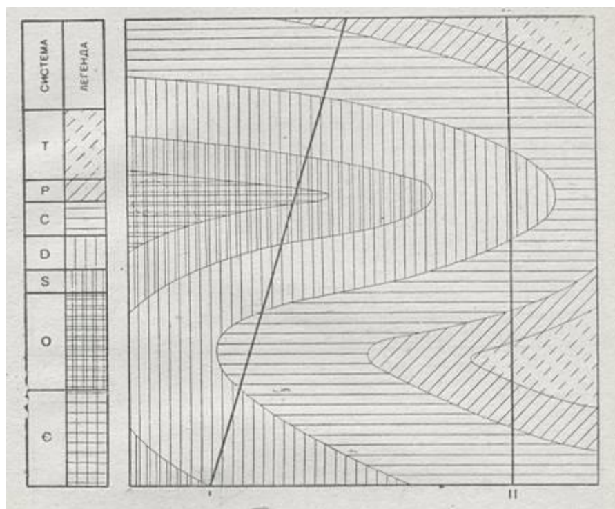
Рис.5. Геологическая карта участка со складчатым залеганием слоев и стратиграфическая колонка к ней (к зад. 6)
