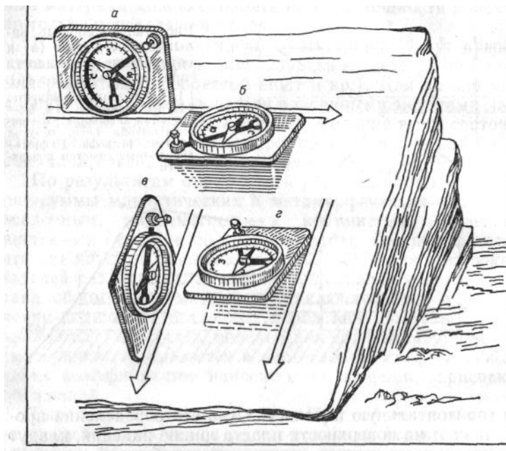
Приемы работы с горным компасом:
