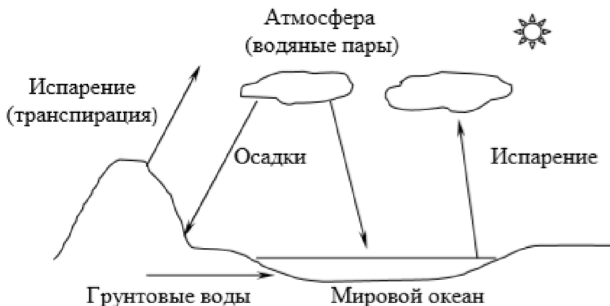
Рис. 5. Схема биогеохимического цикла воды
