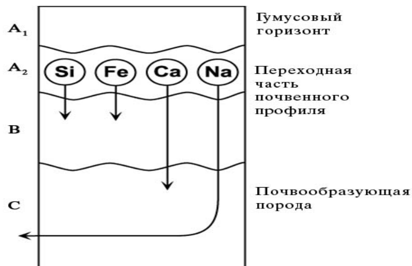
Рисунок - Почвенный профиль автоморфных почв.
