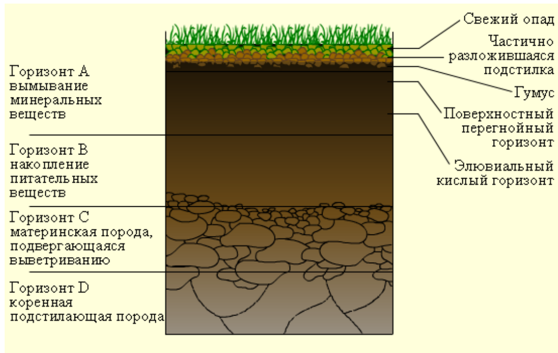
Рисунок - Почвенный профиль
