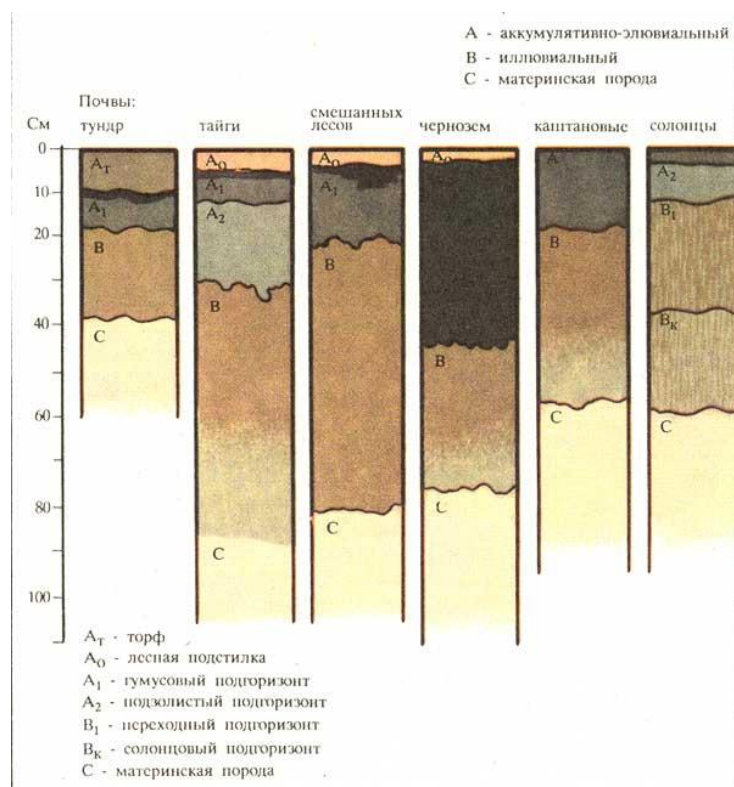
Рисунок – Примеры изображения почвенного профиля
