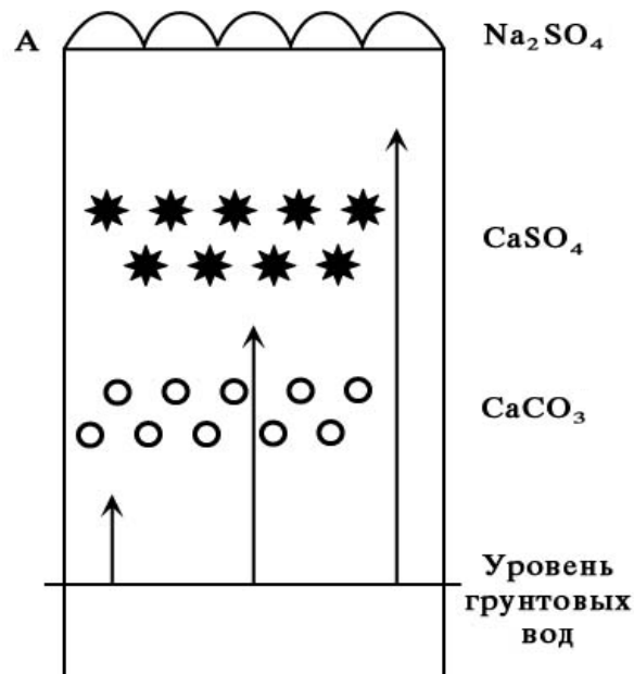
Рисунок - Почвенный профиль гидроморфных почв
