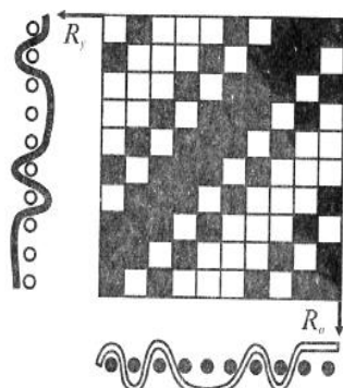
Рис. 28. Сложная саржа
