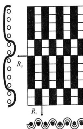
Рис. 24. Репс основной
