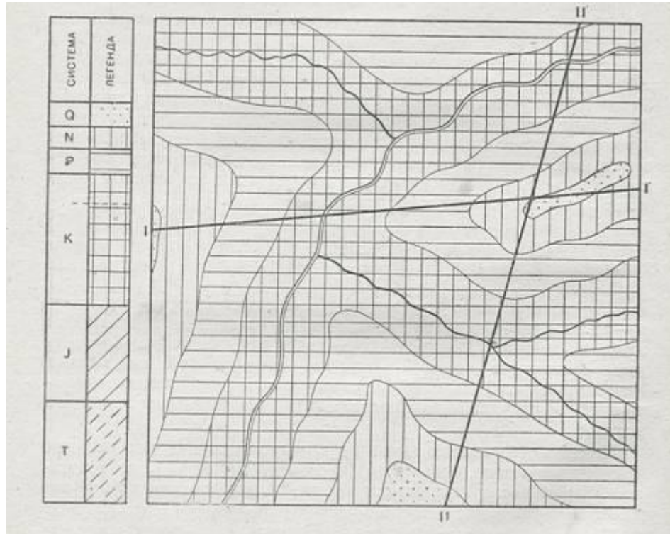
Рис. 2. Геологическая карта территории с горизонтальным залеганием слоев (без топографической основы) и стратиграфическая колонка к ней (к зад. 3)
