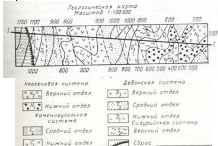
Рис. 14. Геологическая карта
