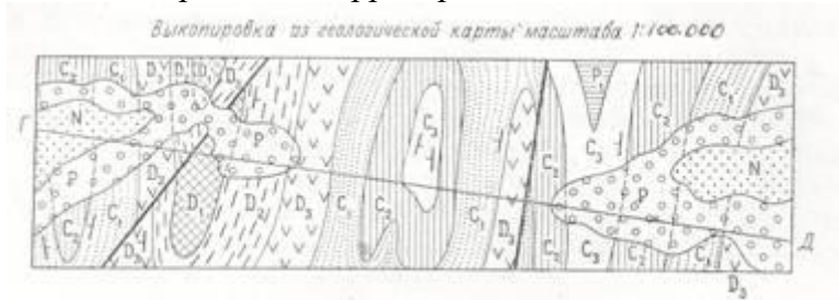
Рис. 13. Фрагмент геологической карты для района со складчатым залеганием горных пород, осложненным сбросами
