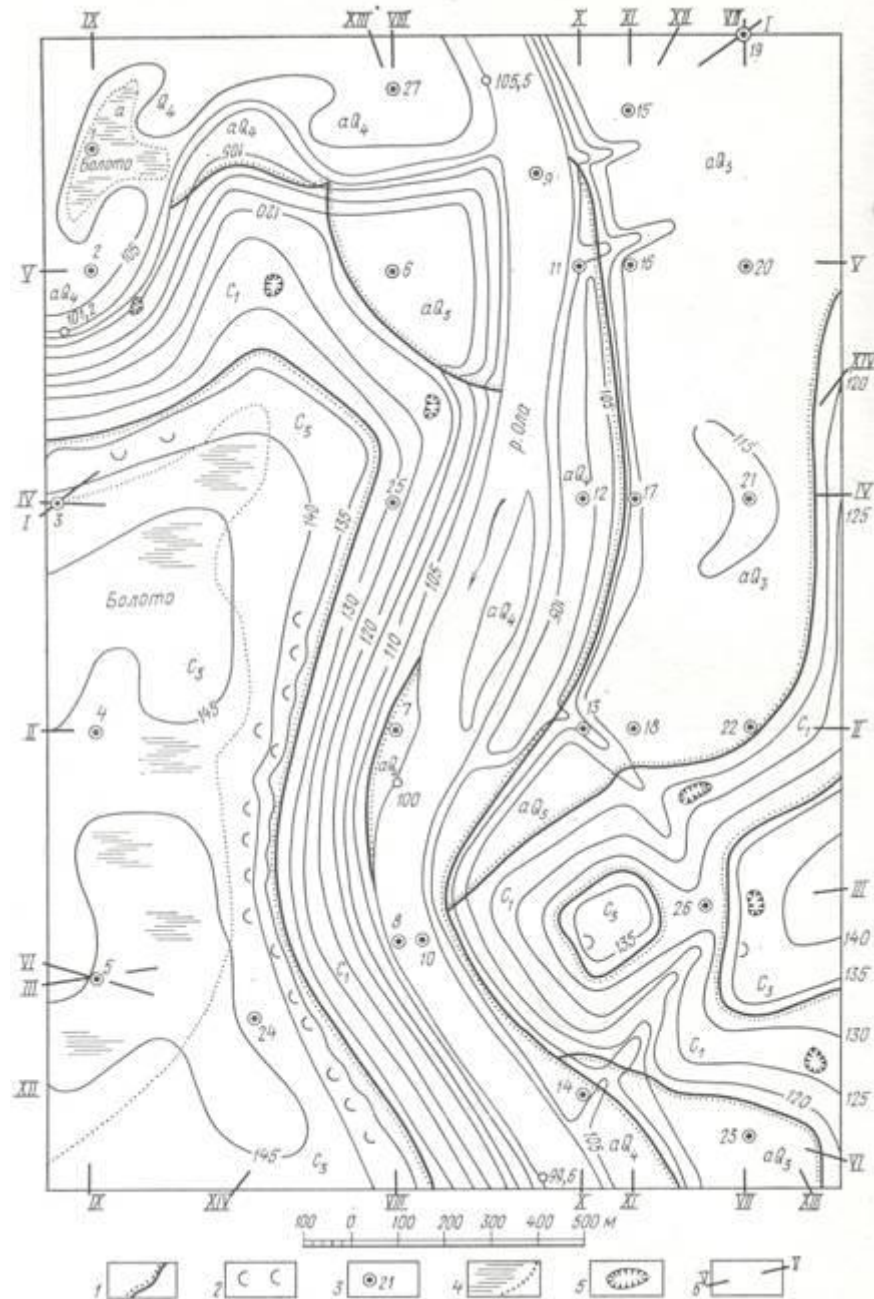
Рис. 16. Геологическая карта:
