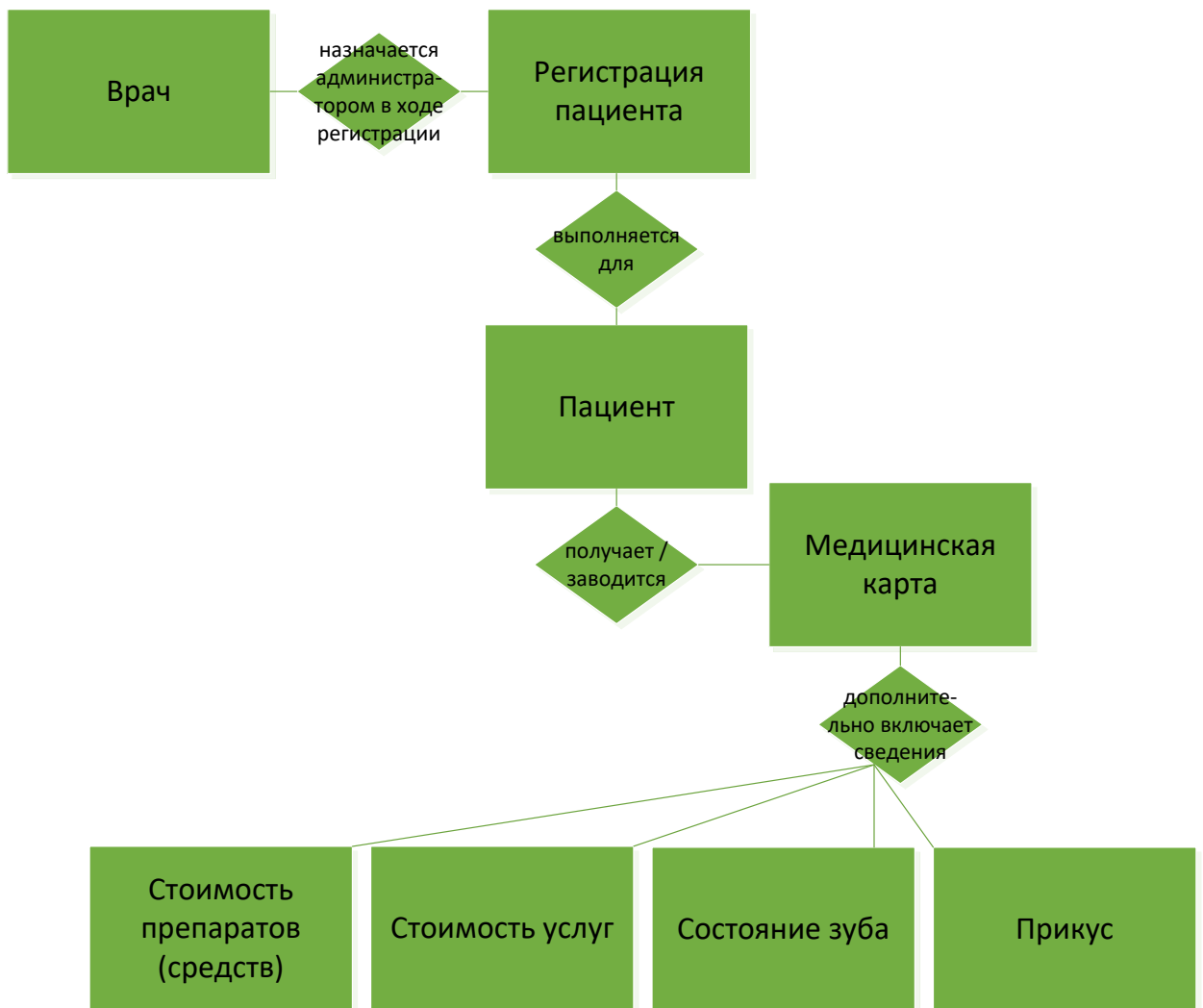
Рис. 13 – Концептуальное проектирование информационной системы в Microsoft Visio (нотация Чена) (модель типа «сущность-связь»)
