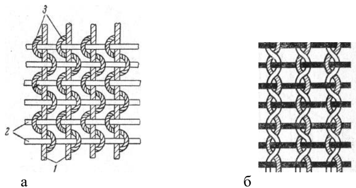
Рис.37. Схема ажурного переплетения: а) ткани на станке: 1 - основные нити; 2 - уточные нити; ажурные (перевивочные) основные нити; б) ткани, снятой со станка КРУПНОУЗОРЧАТЫЕ ПЕРЕПЛЕТЕНИЯ
