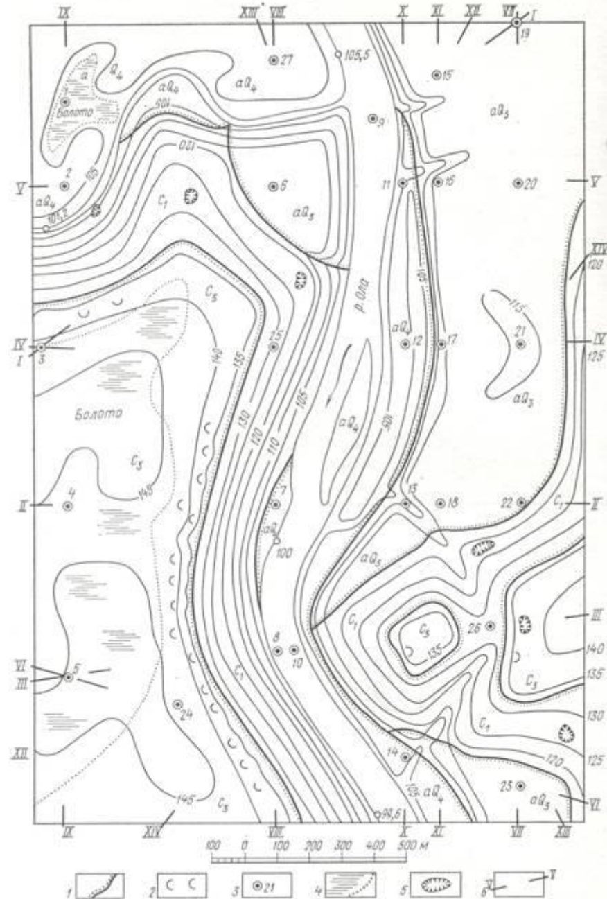
Рис. 16. Геологическая карта:
