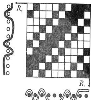
Рис. 28. Сложная саржа
