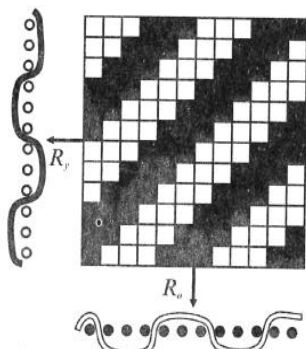
Рис. 27. Усиленная саржа
