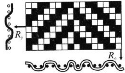
Рис.30. Обратная саржа
