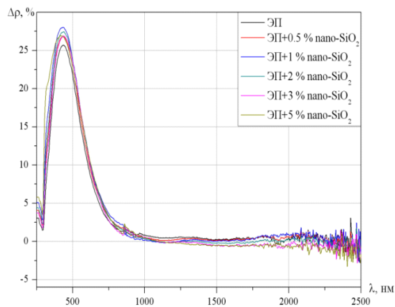
Рисунок 1 – Разностные спектры диффузного отражения ( \Delta\rho = \rho_0 - \rho_\Phi ) кремнийорганического лака (а), лака на основе эпоксидных смол (б) – название рисунка печатается по центру, с заглавной буквы
